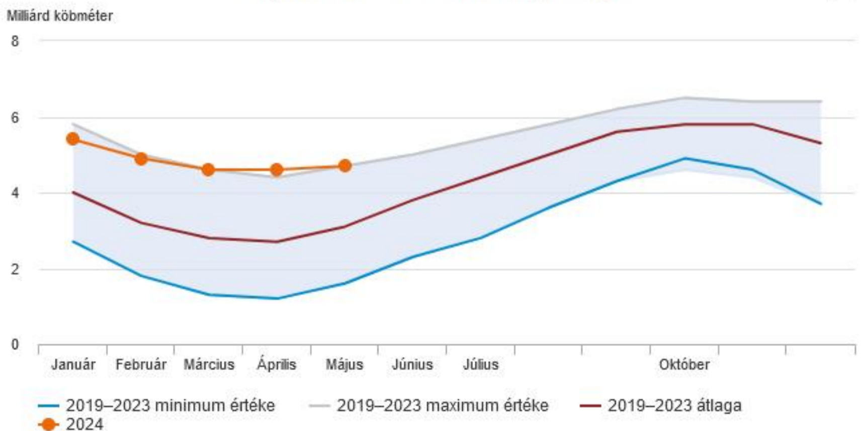
A földgáztárolók készlete az adott hónap 15. napján*
